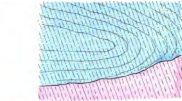
Fig. 5. Überspringen der Schieferung des Gneisses auf den C-förmig gebogenen Kalk am oberen Kalkkeil d. Jungfrau
